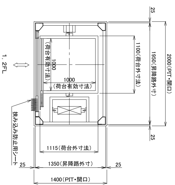
A-A矢視
