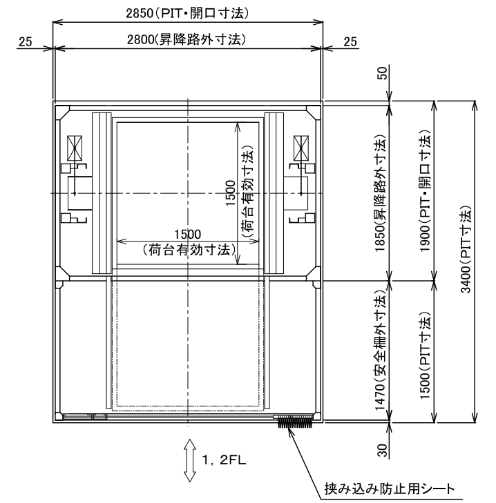
A-A矢視図
