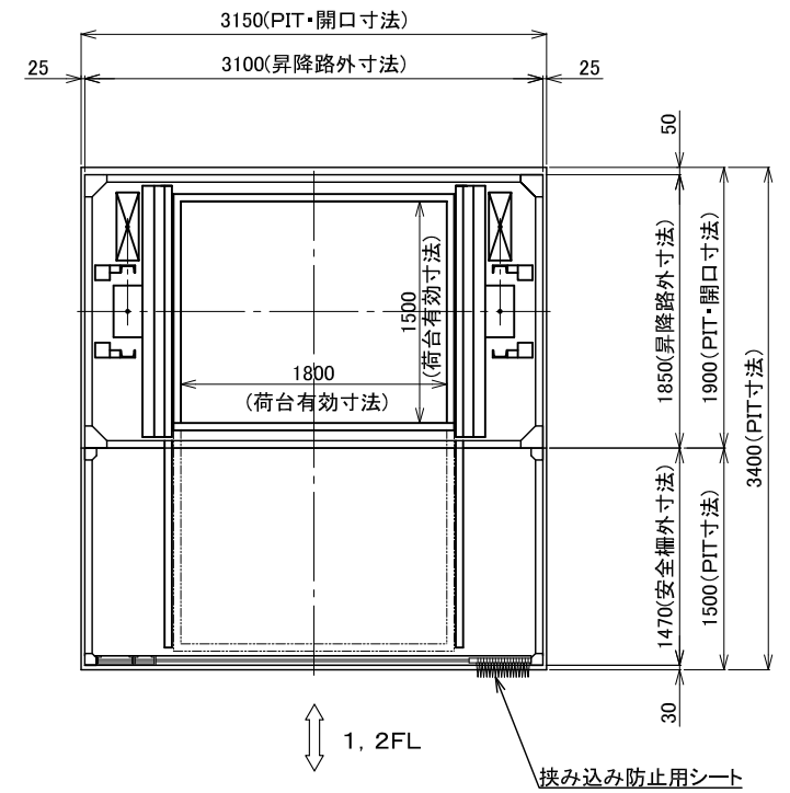
A-A矢視図
