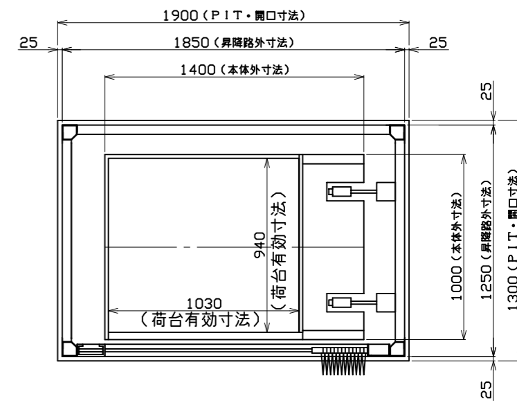
1、2FL A-A矢視図
