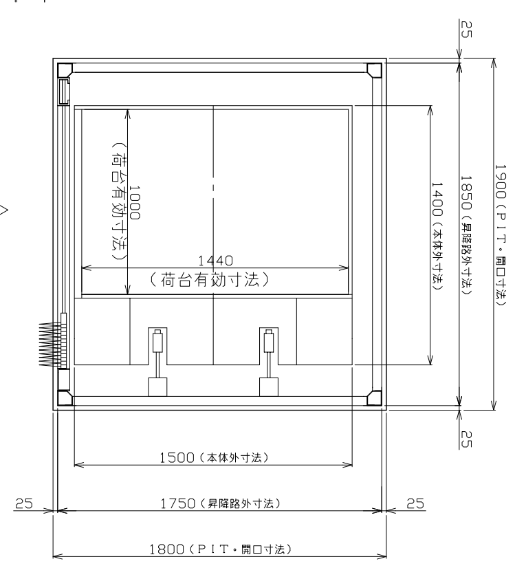
1、2F L A-A矢視図
