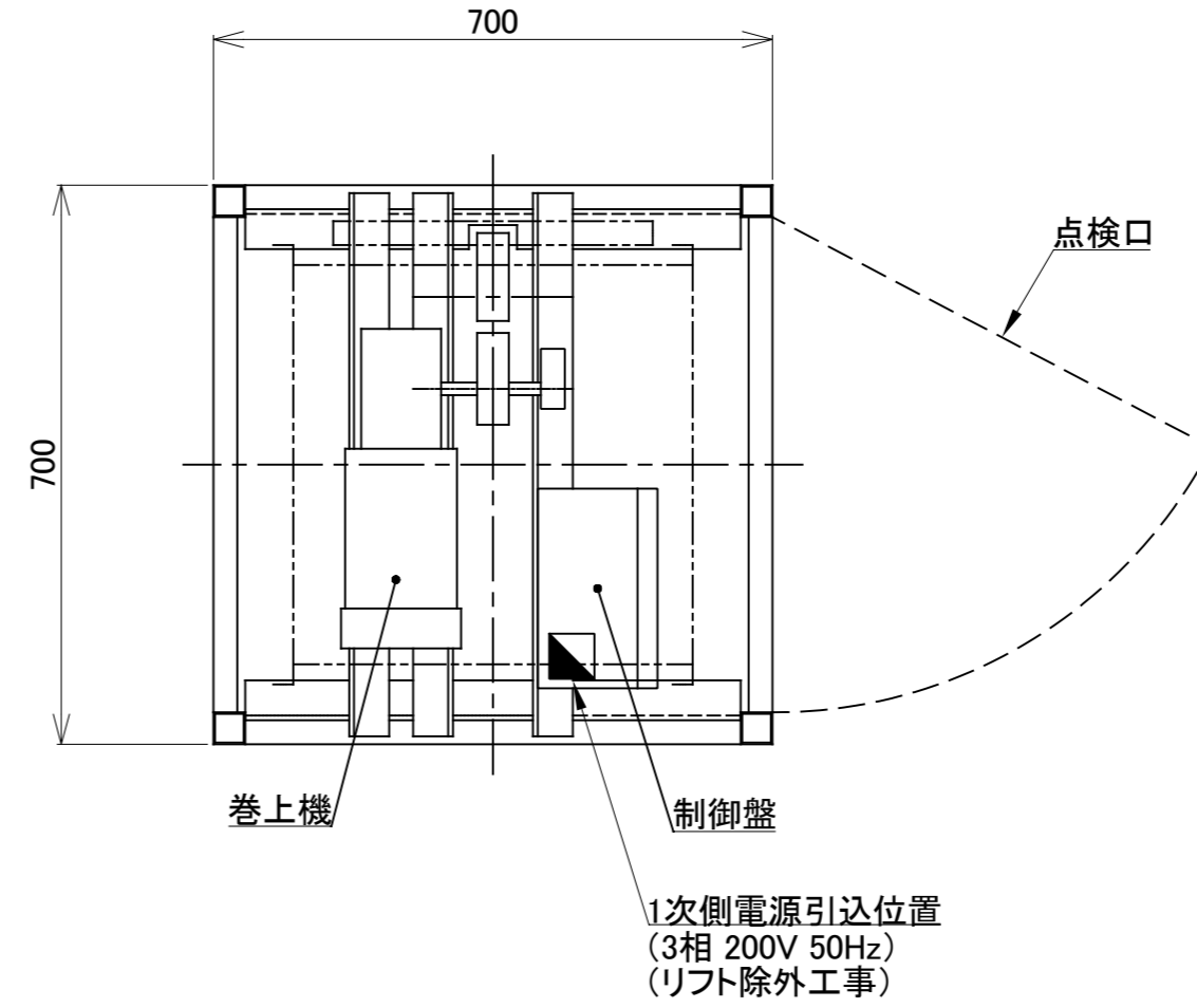
機械室 平面図 S=1/10
