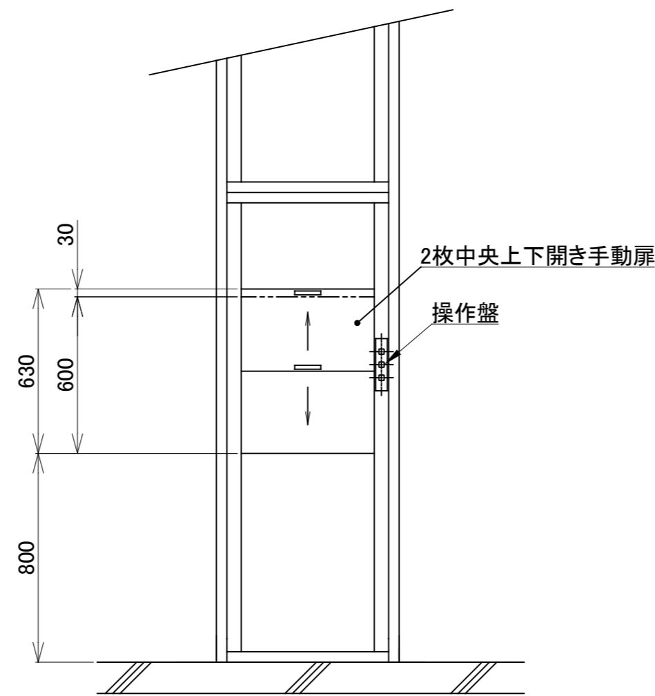
出シ入レロ 立面図
