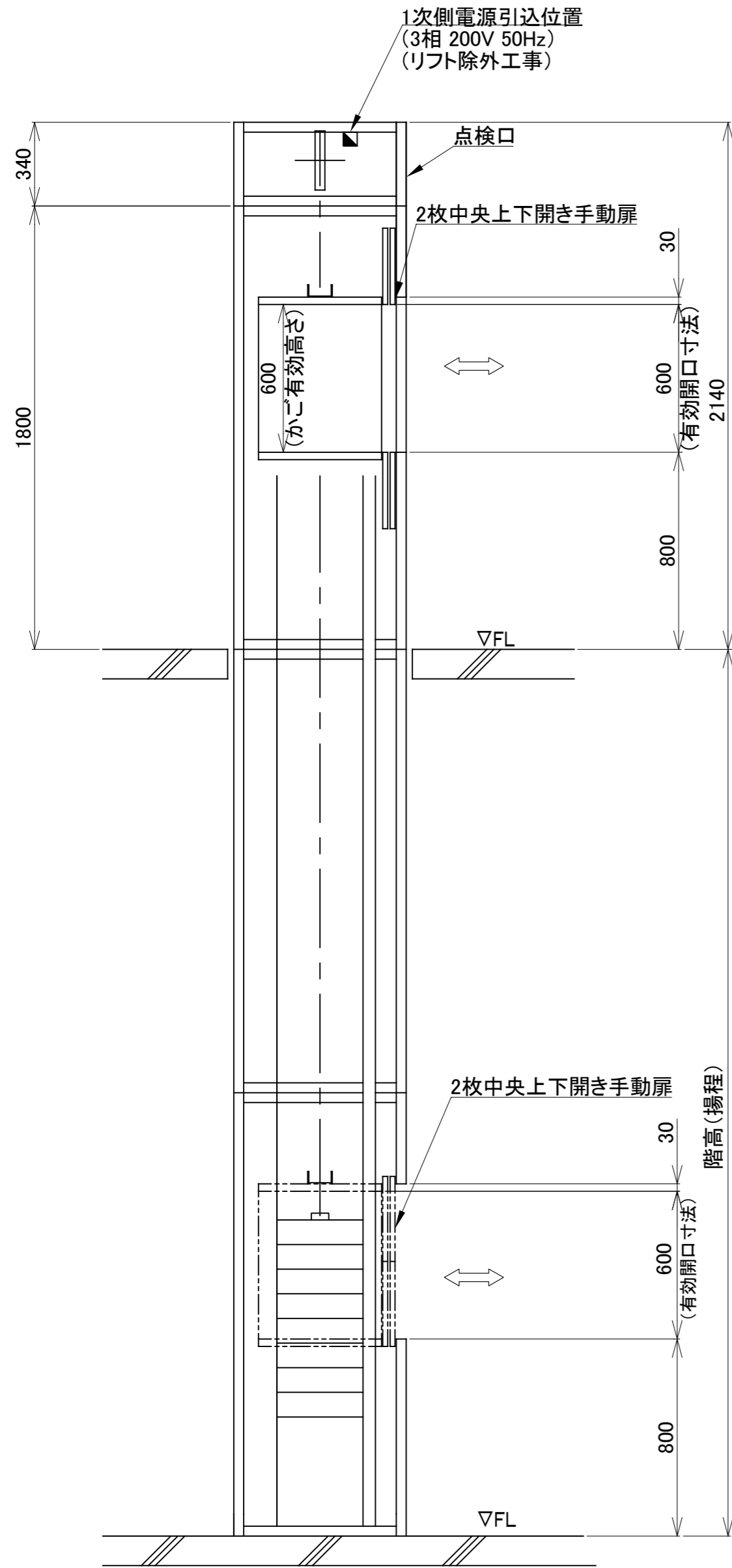
昇降路断面図
