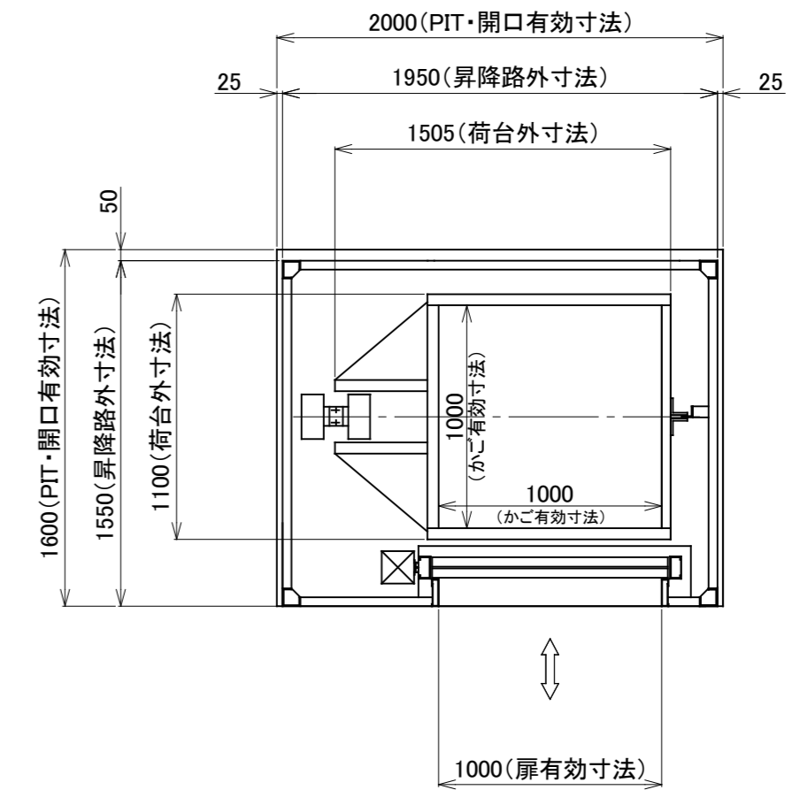
A-A矢視図
