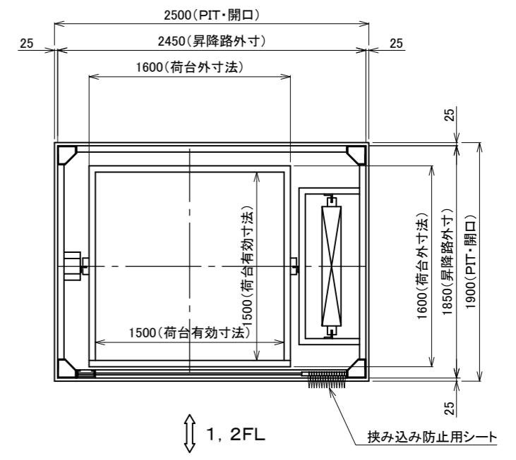
A-A矢視
