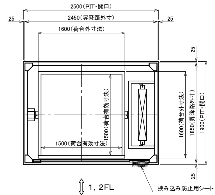
A-A矢視
