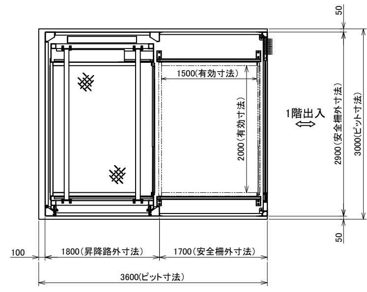
S1-S1 (1F平面)
