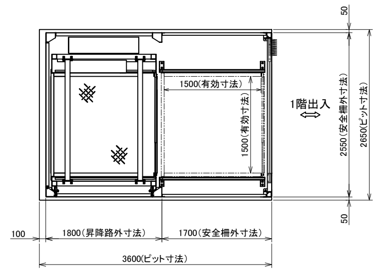
S1-S1 (1F平面)
