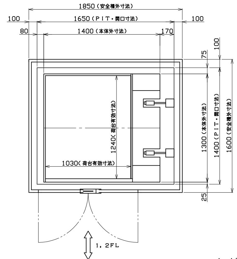
A-A矢視図
