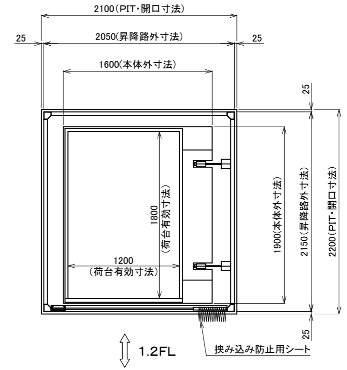
A-A矢視図
